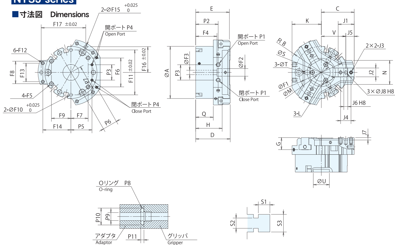
ベース配管詳細 Detail of direct connecting
