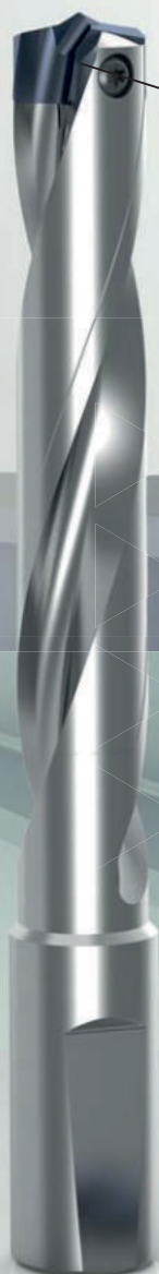
Wechselplattenhalter Multiplex HPC Art.-Nr. 86684
