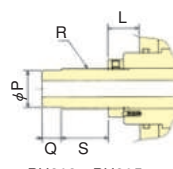
PU203~PU205 (ドローバー接続部)
