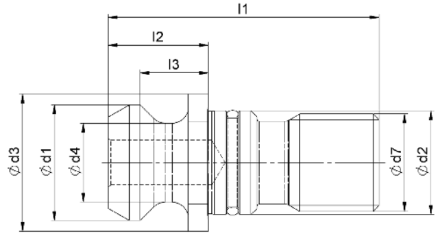
Anzugsbolzen DIN ISO 7388-3 UF (ISO 7388-2 Form B)
